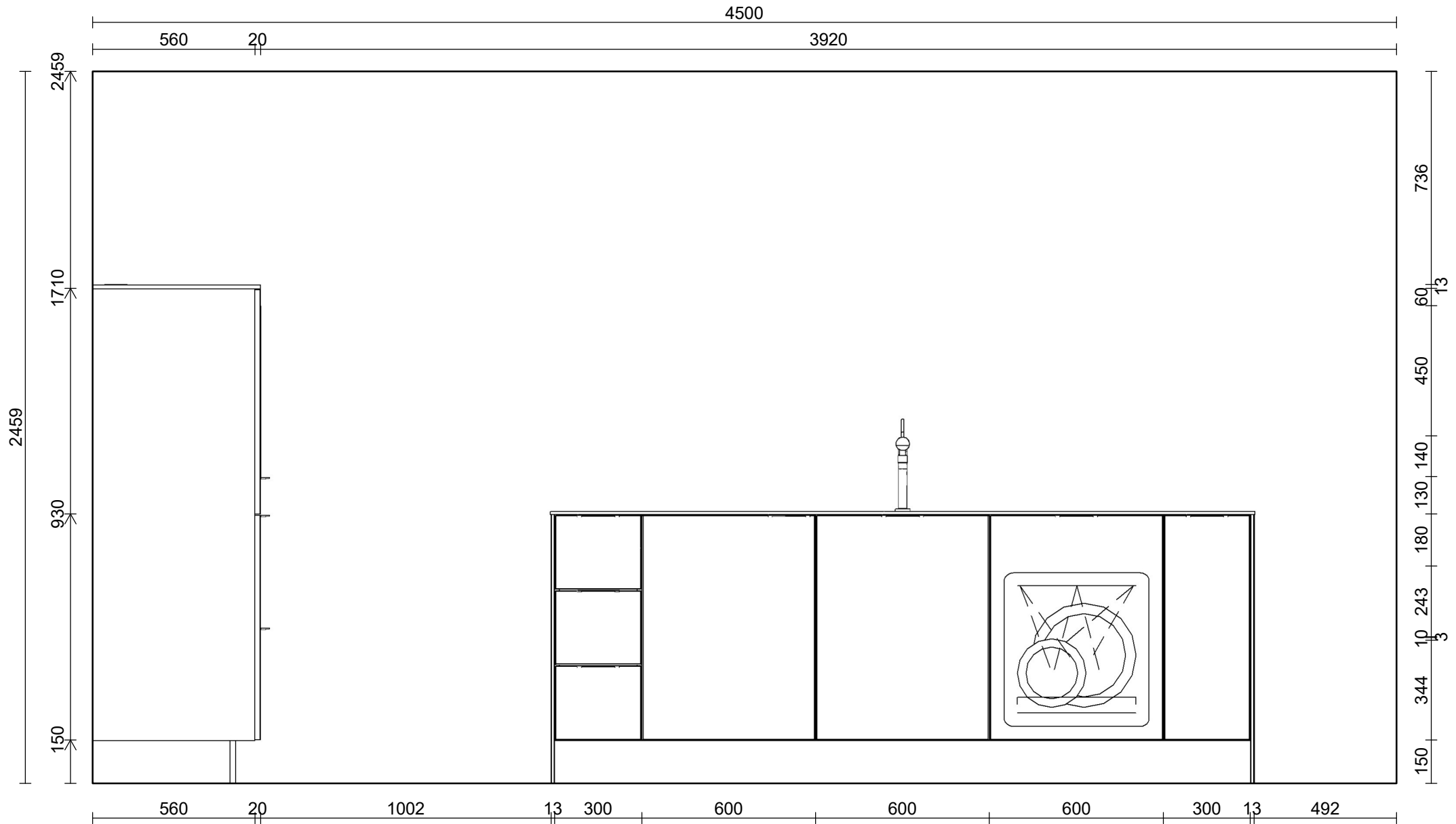
Wand - 7 / Masstab: Angepasst
