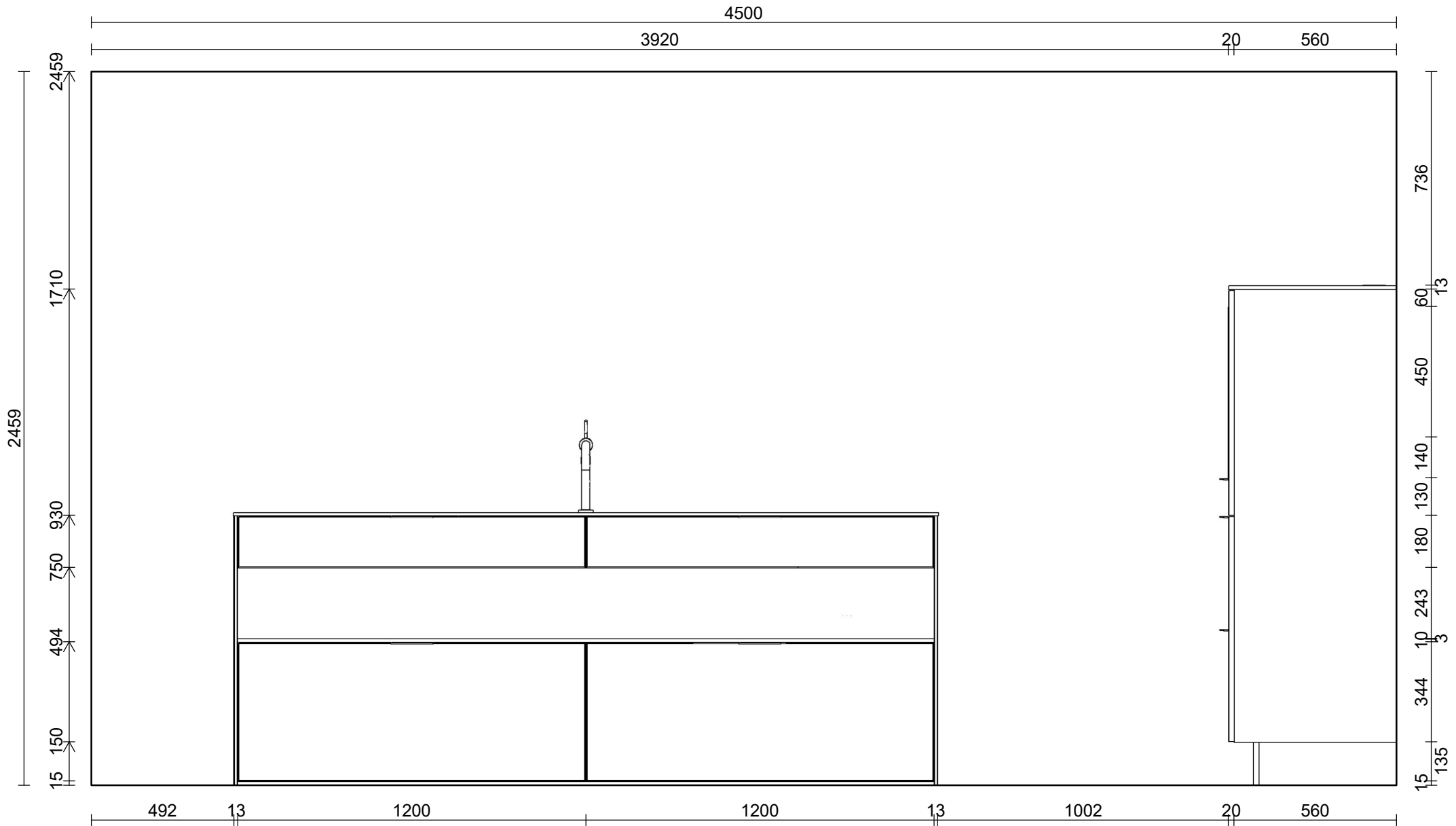
Wand - 8 / Masstab: Angepasst
