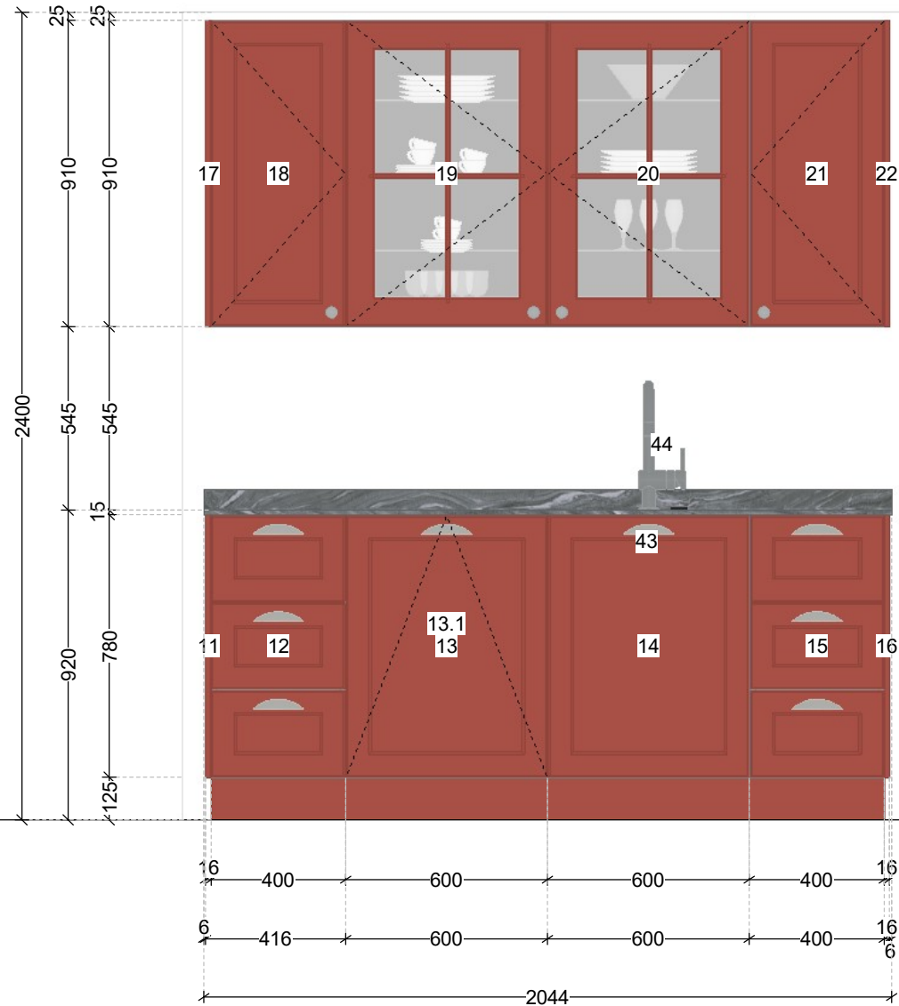
Wand - 72 / Massstab: 1:20 (A4)
